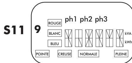
Contrôle du fonctionnement de l'afficheur (usage gestionnaire du réseau de distribution)
