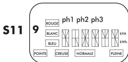
Contrôle du fonctionnement de l'afficheur (usage gestionnaire du réseau de distribution ) L'affichage varie suivant la marque
